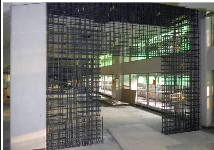
2階ロビー耐震補強工事（鉄筋取り付け）
